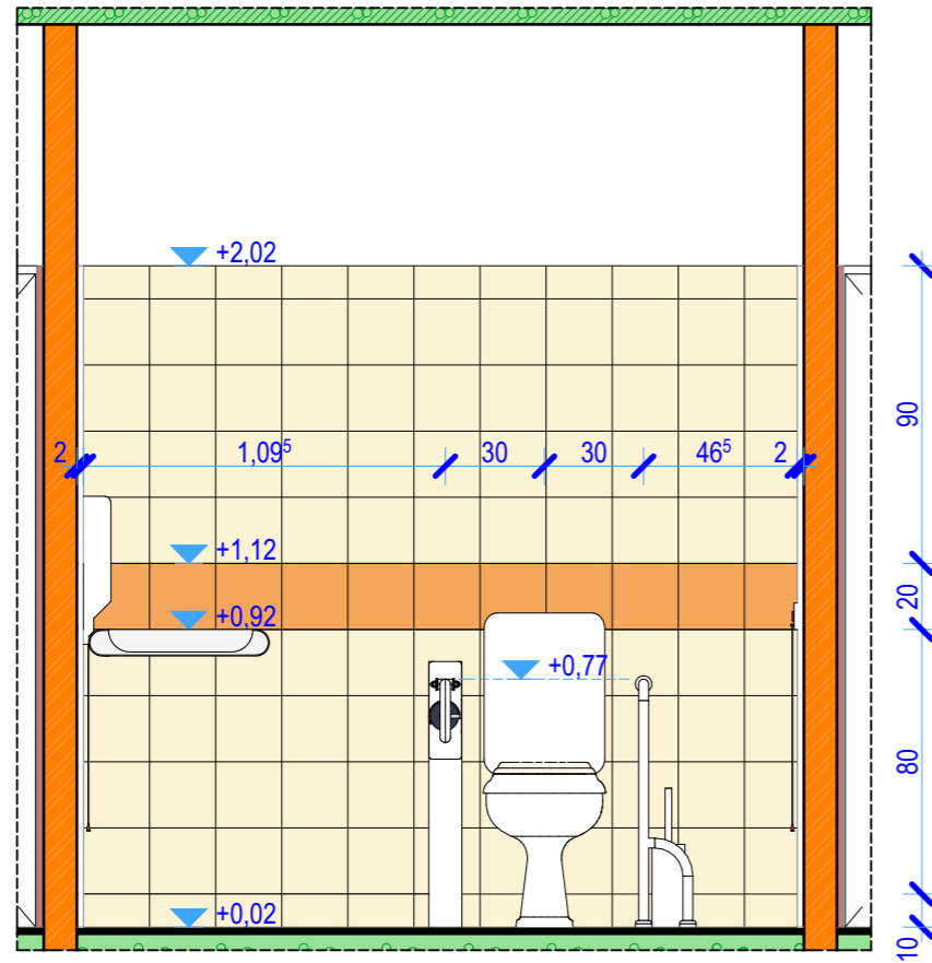
F-03 Falnézet 3 1:25
