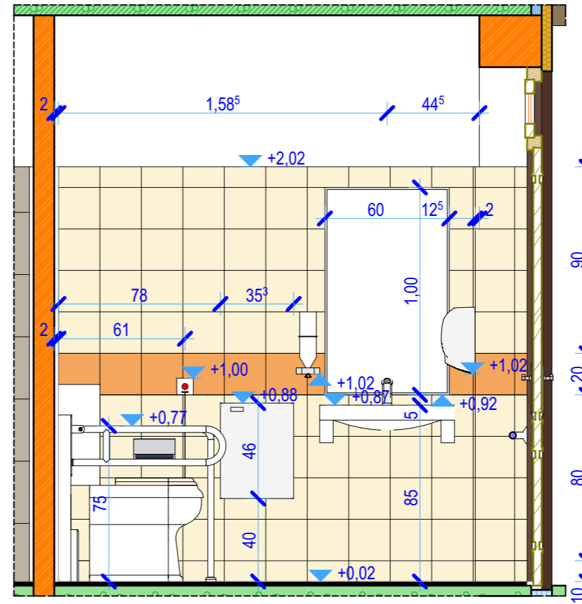
F-04 Falnézet 4 1:25
