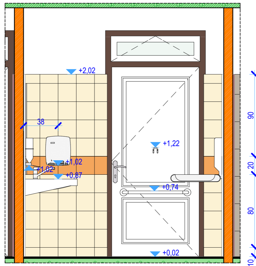
F-03 Falnézet 3 1:25
