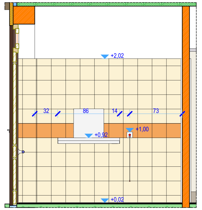
F-04 Falnézet 4 1:25
