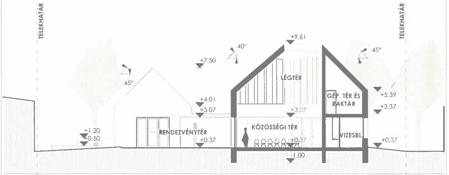
B-B METSZET
