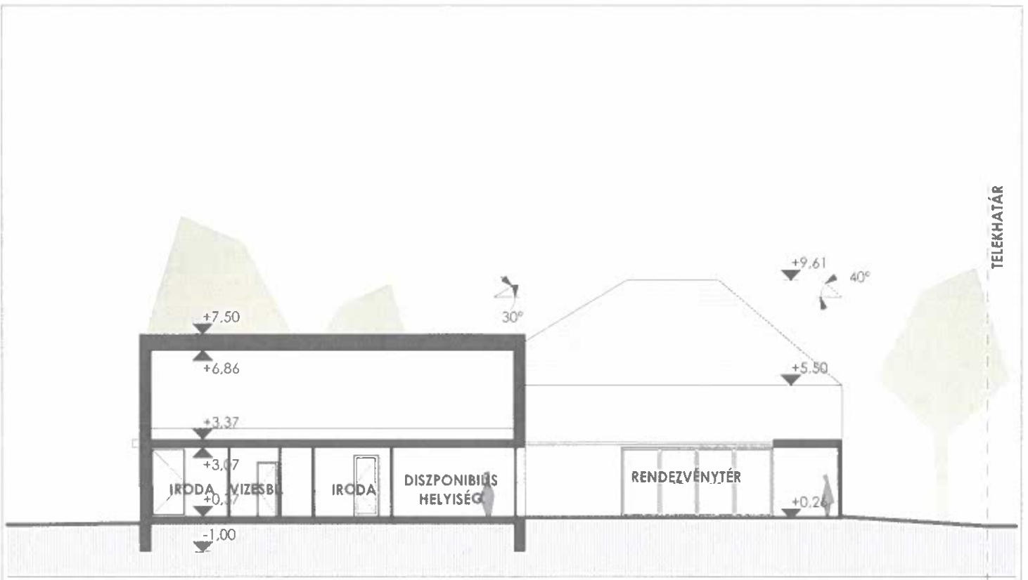
A-A METSZET
